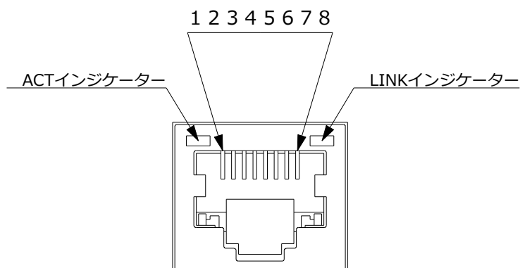
SL-C シリーズ RJ-45
