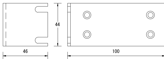
○本体連結用金具 (前面)
