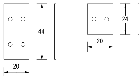
○本体連結用金具 (前面)
